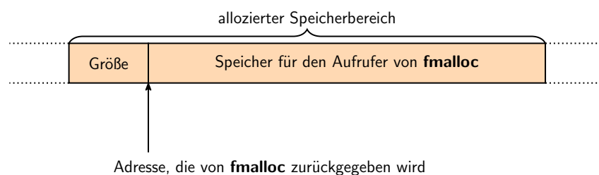
Abbildung 2: Reservierter Speicherbereich mit dazugehöriger Größe.
