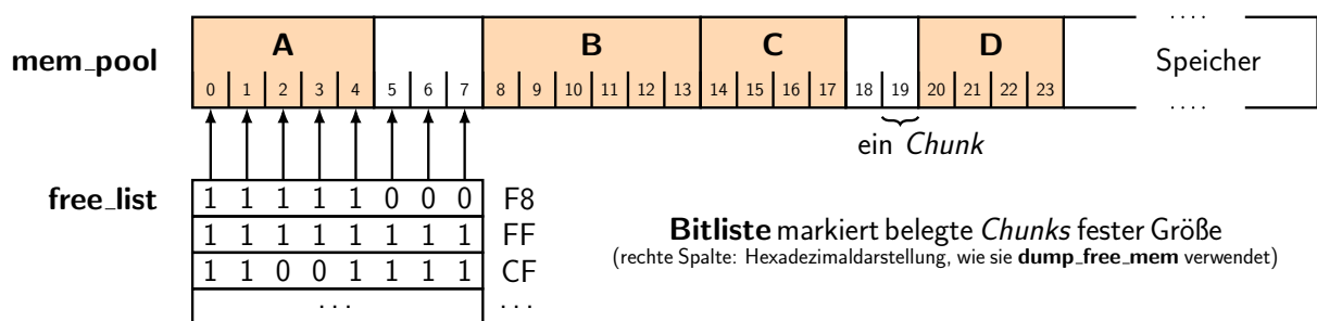
Abbildung 1: Freispeicher-Bitliste mit zugehörigen Chunks fester Größe (z.B. 32 Bytes) im Speicher.
